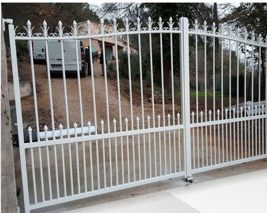
► Portail battant Vitry modifié, traverse haute en forme CDG avec fers-de-lance n°4, avec rangée de petites volutes. Soubassement avec double barreaudage comprenant rangée de fers-de-lance dans la traverse intermédiaire. Sabot de sol métallique en option.
